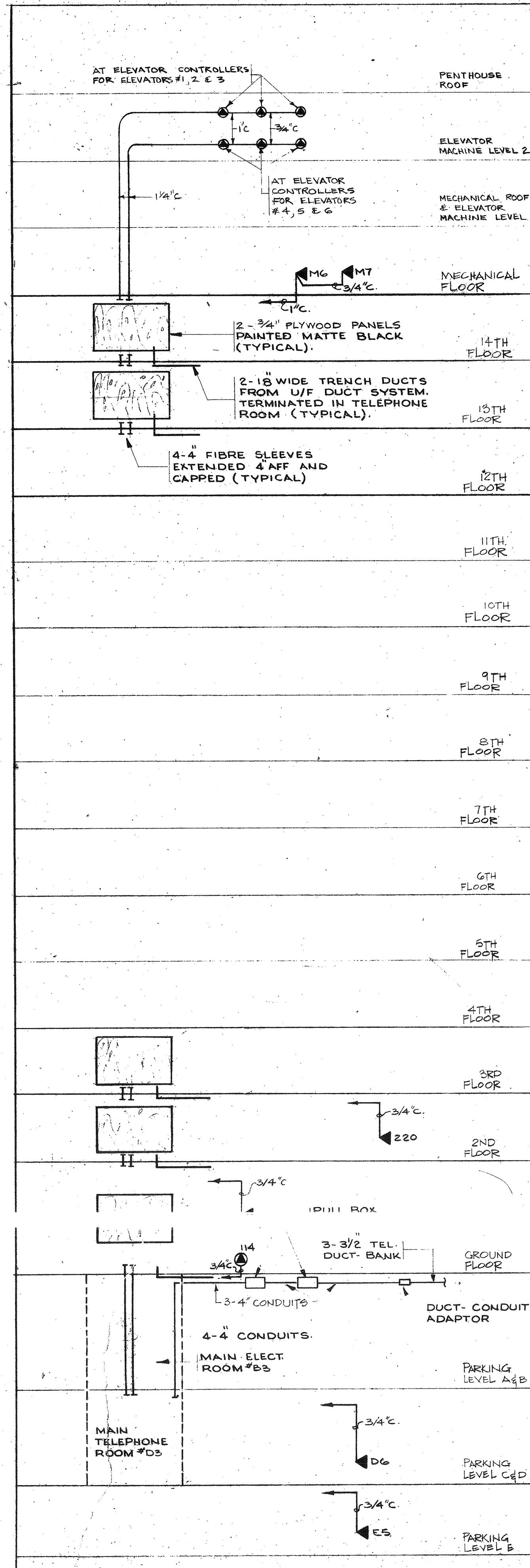
3 TELEPHONE SYSTEM RISER N.T.S.
