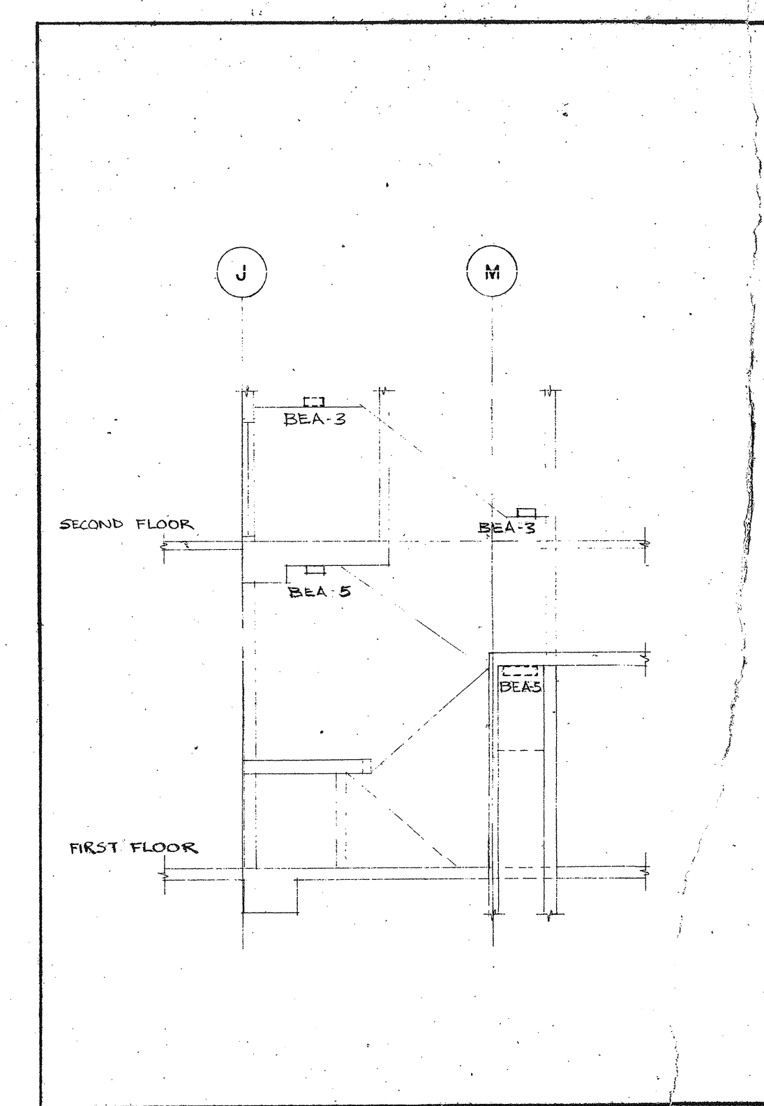
5 STAIR S5 LIGHTING RISER SCALE: 1/8"=1'-0"
