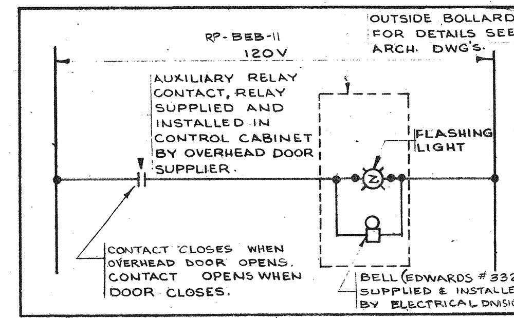
20 SCHEMATIC #19
