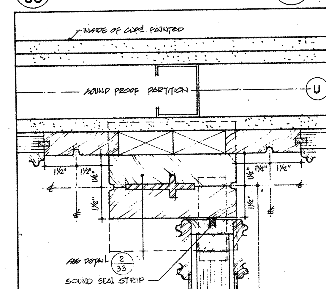
7/33 PLAN
