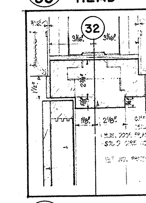
30/33 DOOR HEAD
