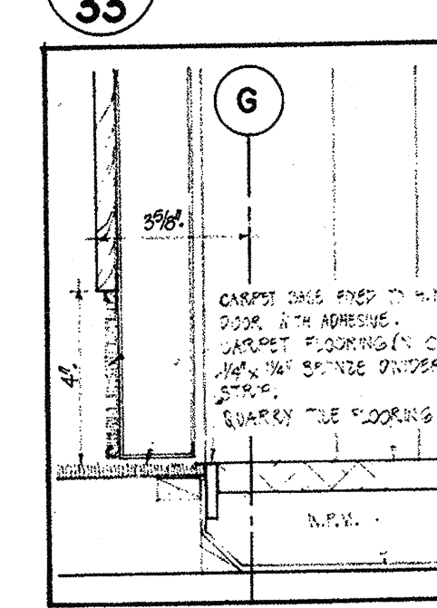
28/33 DOOR SILL
