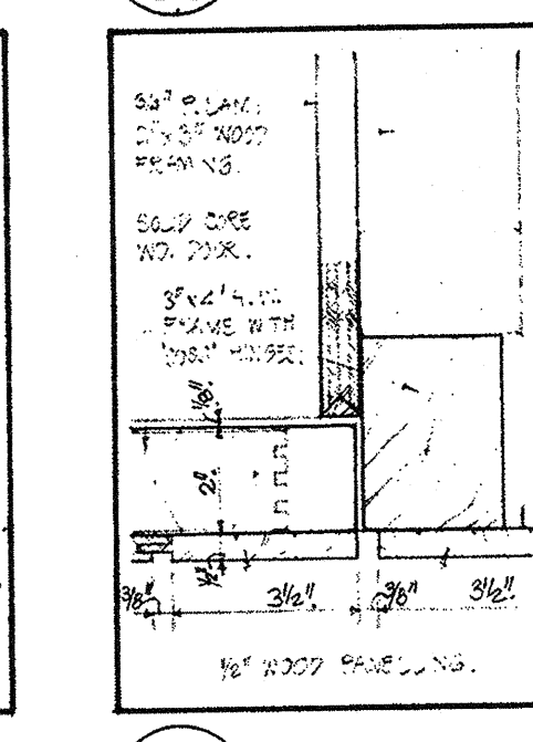
31/33 DOOR JAMB
