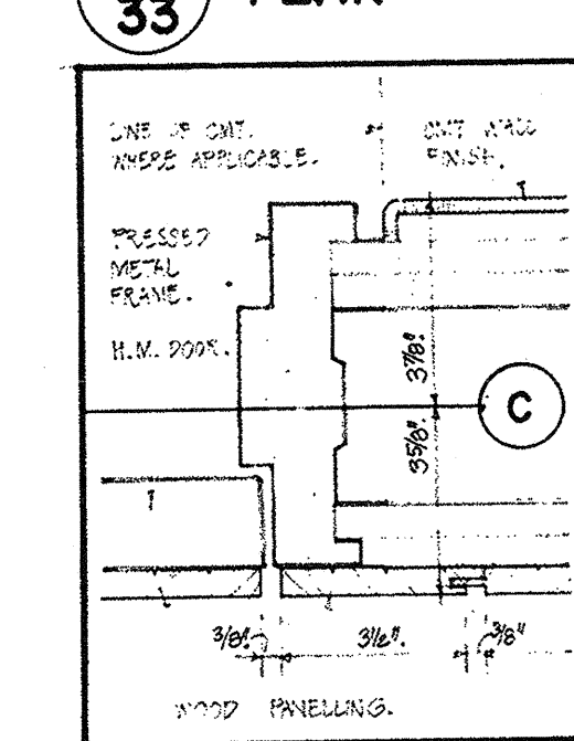
27/33 DOOR JAMB
