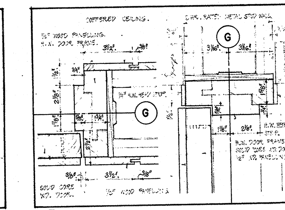
25/33 DOOR JAMB & HEAD
